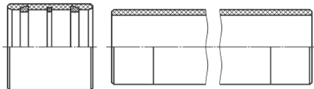
Рисунок 8 — Раздельная комплектация труб и муфт
