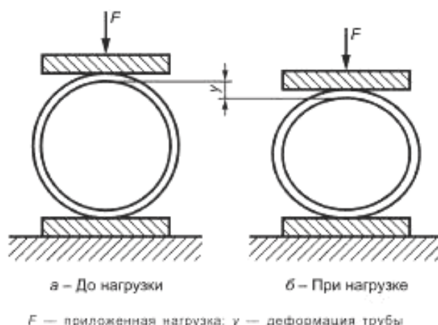
Рисунок 10 — Схема испытания на нагрузочной машине
