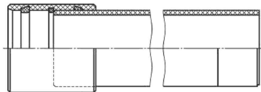
Рисунок 7 — Комплектация трубы с муфтой на уплотнителях
